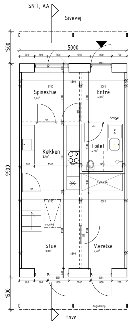
01 STUEETAGE MÅL 1:100
