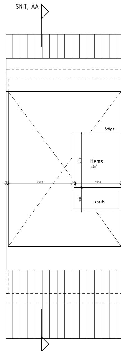
02 HEMS MÅL 1:100
