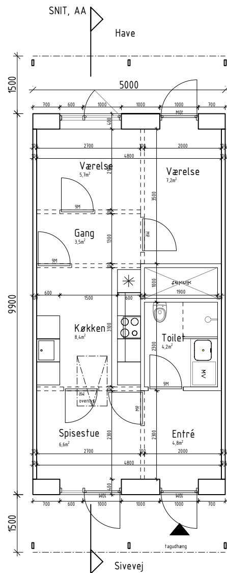
01 STUEETAGE MÅL 1:100
