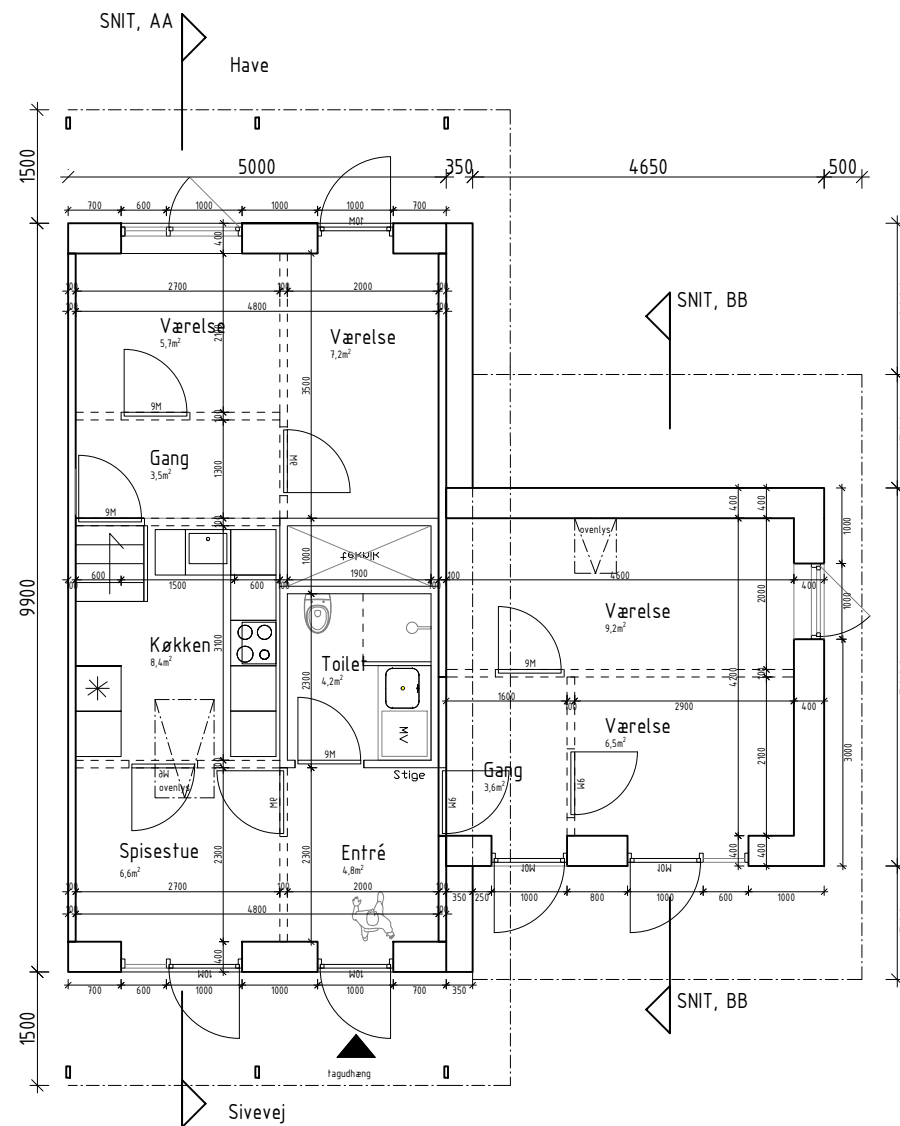
01 STUEETAGE MÅL 1:100
