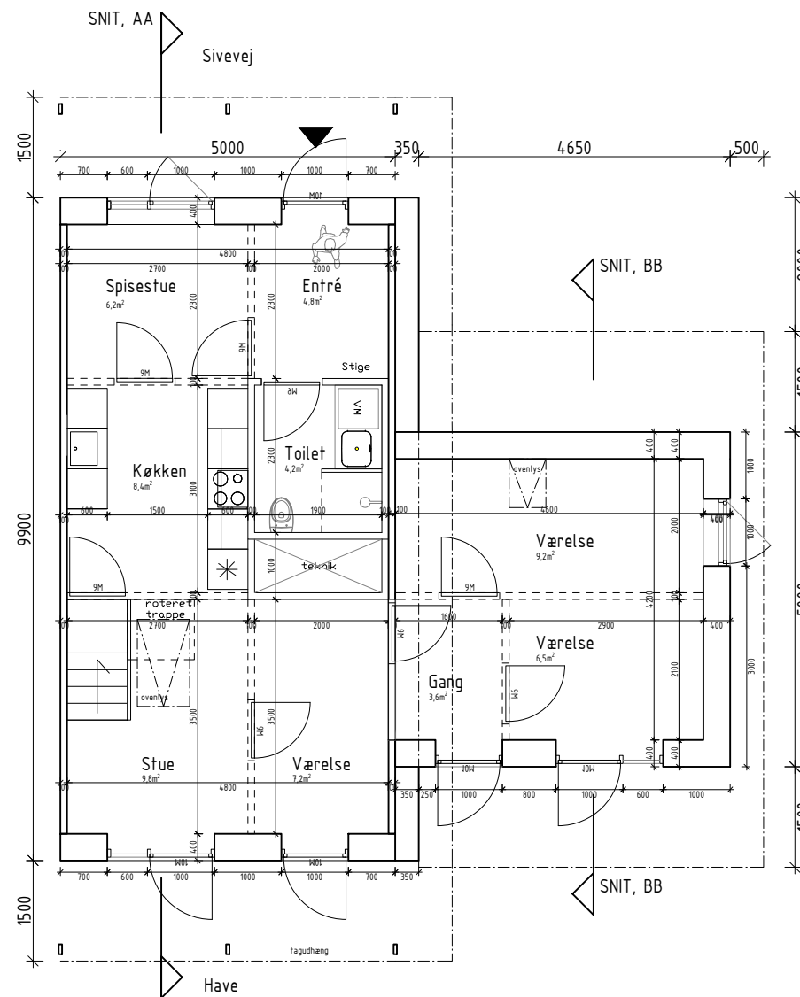
01 STUEETAGE MÅL 1:100
