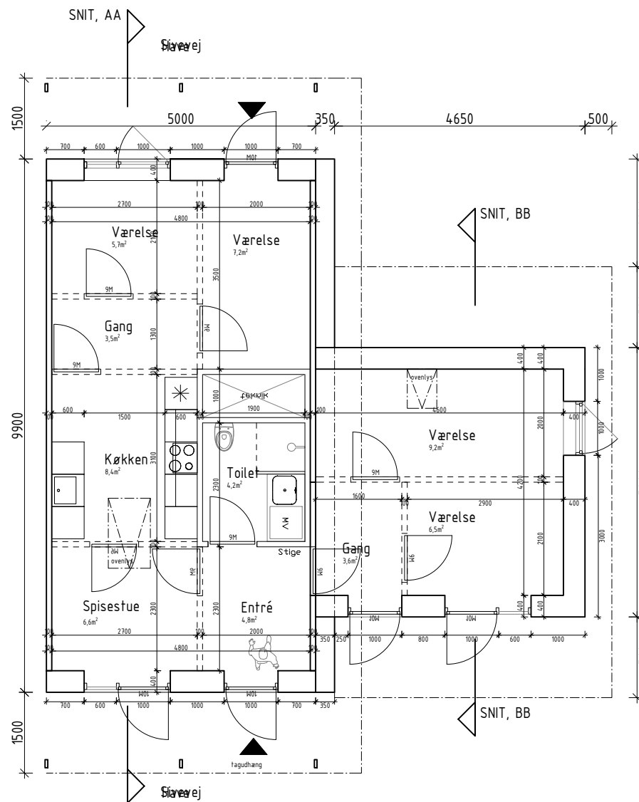
01 STUEETAGE MÅL 1:100
