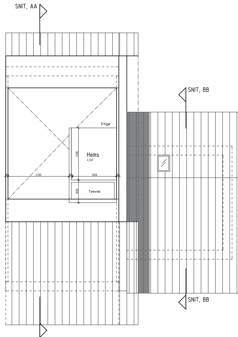
02 HEMS MÅL 1:100
